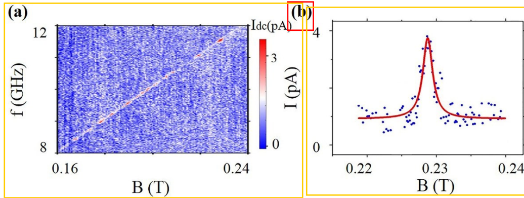
图 3.7 (a) 漏电流随微波频率和外加磁场的演化,呈现出线性关系。(b) 在微波频率为 11.5 GHz、功率为 -11.5 dBm 时对共振峰进行高斯拟合(红色曲线)。
