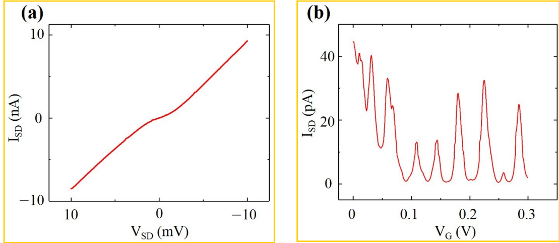
图 2.11 (a) 量子点输运电流随源漏偏压 V_{SD} 变化的 I-V 曲线图。(b) V_{SD} = 0.5 \text{ mV} 时量子点的库伦振荡曲线。
