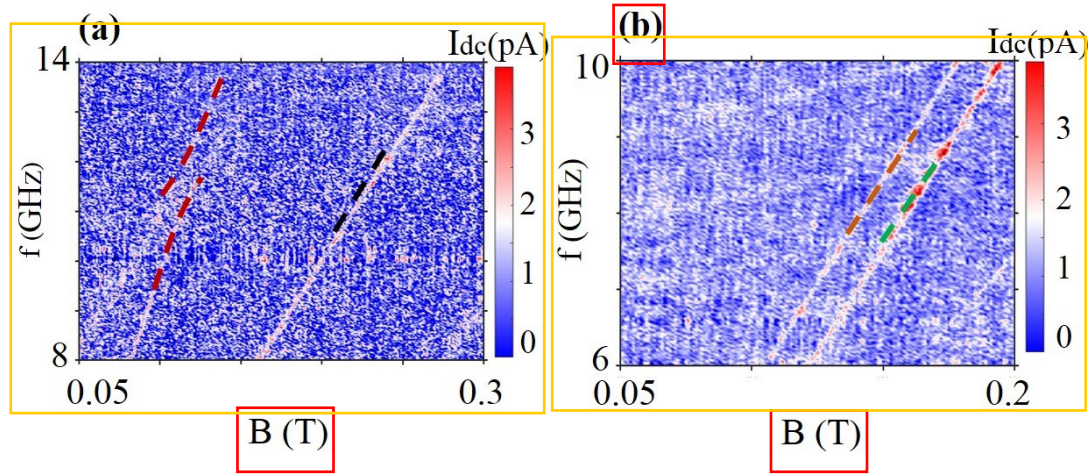
图 3.8 (a) 在 V_{G3} = -0.05 V 时漏电流随微波频率和外加磁场的演化，观测到多条不同模式下的电偶极自旋共振谱线，分别用红色虚线和黑色虚线标注。(b) 与(a)相同区域，中间栅极电压 V_{G3} 从 -0.05 V 调节到 -0.048 V。观测到两条斜率相似的谱线，分别用棕色虚线和绿色虚线标注。
