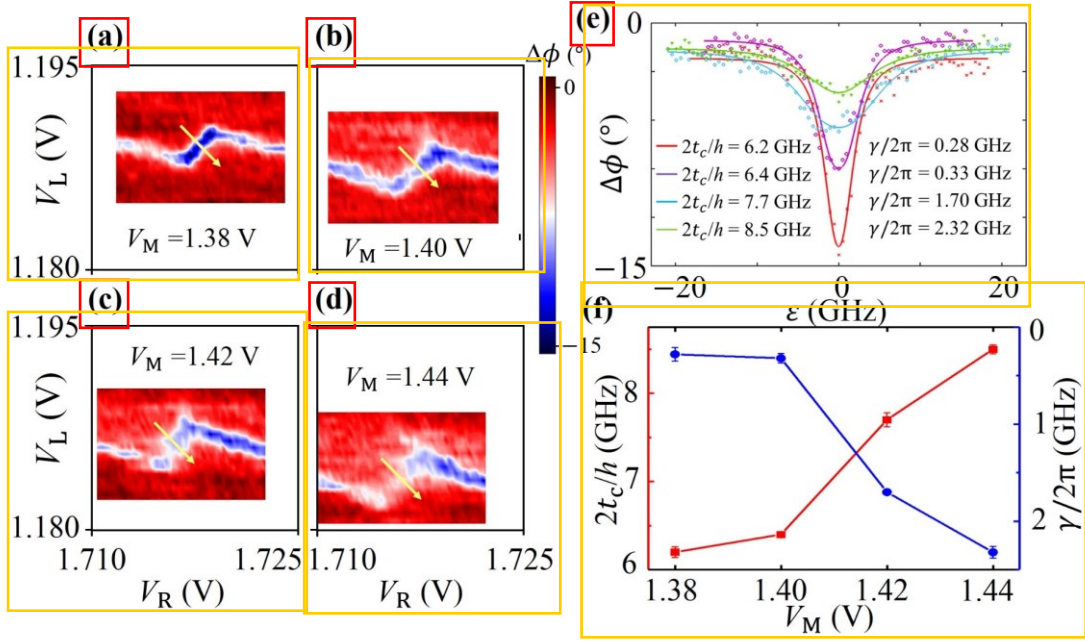
图 4.8 (a)-(d) 不同中间栅极电压 V_M 下, 点间隧穿区域相位变化的电荷稳定性相图, 黄色箭头的方向表示沿着失谐线的方向。(e) 不同中间栅极电压下沿着失谐线提取的相位变化, 并分别用公式 4.7 拟合。拟合结果为 [2t_C/h, g_C/2\pi, \gamma/2\pi] = [6.2 \text{ GHz}, 15.0 \text{ MHz}, 0.28 \text{ GHz}] ( V_M=1.38 \text{ V} ), [2t_C/h, g_C/2\pi, \gamma/2\pi] = [6.4 \text{ GHz}, 14.5 \text{ MHz}, 0.33 \text{ GHz}] ( V_M=1.40 \text{ V} ), [2t_C/h, g_C/2\pi, \gamma/2\pi] = [7.7 \text{ GHz}, 16.6 \text{ MHz}, 1.70 \text{ GHz}] ( V_M=1.42 \text{ V} ), [2t_C/h, g_C/2\pi, \gamma/2\pi] = [8.5 \text{ GHz}, 17.8 \text{ MHz}, 2.32 \text{ GHz}] ( V_M=1.44 \text{ V} )。 (f) 隧穿率 2t_C/h 和退相干率 \gamma/2\pi 对应于不同中间栅极电压 V_M 下绘制的曲线图。
