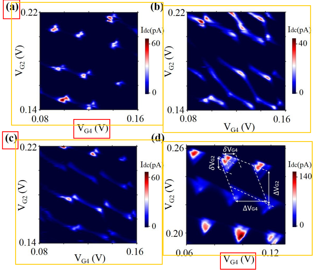
图 3.2 (a)-(c) 当 V_{SD} = 0.5 \text{ mV} , V_{G1} = -0.82 \text{ V} , V_{G5} = -0.2 \text{ V} 时, 在不同中间栅极电压 V_{G3}(0 \text{ V}, -0.02 \text{ V}, -0.04 \text{ V}) 下, 扫描 V_{G2} 和 V_{G4} 测到的输运相图。(d) 当 V_{SD} = 2 \text{ mV} , V_{G1} = -0.82 \text{ V} , V_{G3} = 0.008 \text{ V} , V_{G5} = -0.17 \text{ V} 时, 观测到一组排列整齐的偏压三角形输运相图。
