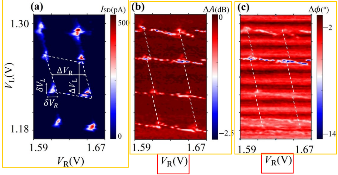
图 4.6 (a) 源漏偏压 V_{SD} = 1.5 \text{ mV} 时，双量子点直流运输的电荷稳定性相图，空穴在量子点中和源漏之间隧穿用白色虚线表示。 \delta V_L 和 \delta V_R 对应偏压三角形的尺寸， \Delta V_L 和 \Delta V_R 表示在左点和右点增加或者删减一个空穴时，左右栅极电压的变化量。(b)和(c)分别对应着相同栅极电压范围内的幅值和相位变化相图
