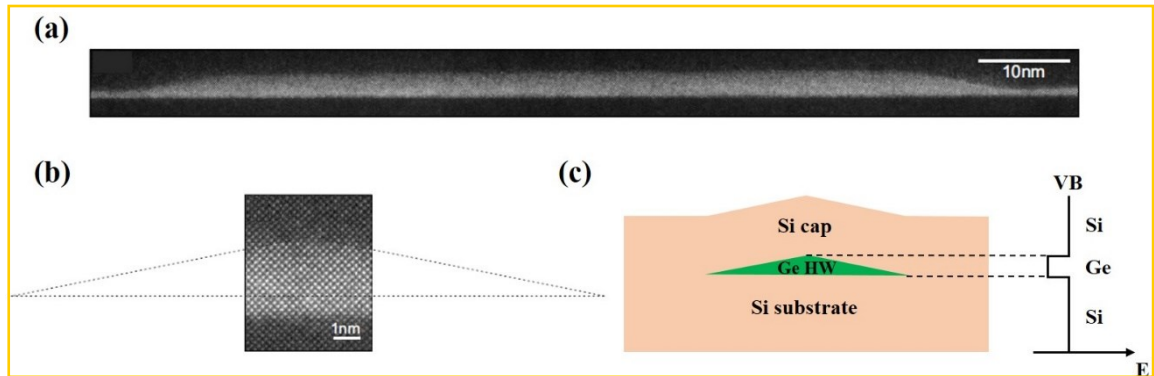
图 2.3 (a) Ge 纳米线径向截面的扫描透射电子显微镜图，图片引自[5]。(b) Ge 纳米线横截面的扫描透射电子显微镜图，虚线部分表示纳米线的形状，图片引自[5]。(c) Ge 纳米线的能带结构示意图。
