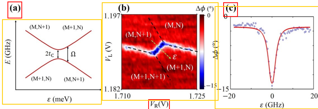
图 4.7 (a) 双量子点沿着失谐量方向的能级结构表示为 \Omega = \sqrt{(2t_c)^2 + \varepsilon^2} ，在失谐量 \varepsilon = 0 时，有一个最小能级劈裂 2t_c 。(b) 空穴在 (M, N+1) \leftrightarrow (M+1, N) 点间区域隧穿时相位变化的电荷稳定性相图，绿色箭头的方向表示沿着失谐量的方向。(c) 蓝色圆点为沿着失
