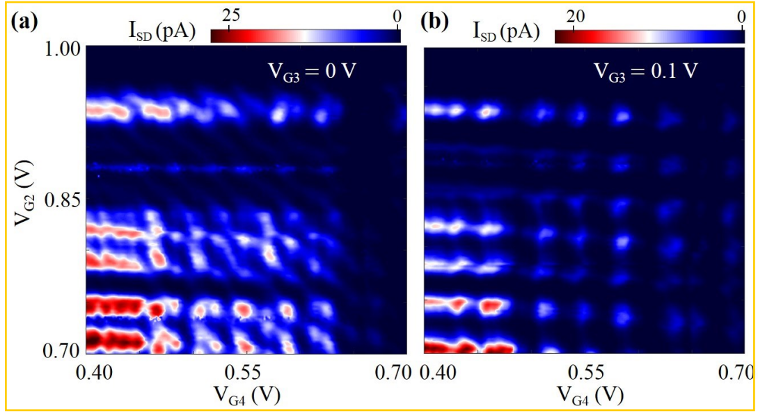
图 2.13 (a) V_{SD} = 0.5 \text{ mV} , V_{G1} = V_{G5} = 0.5 \text{ V} , V_{G3} = 0 \text{ V} 时双量子点的蜂窝图。(b) 和(a) 相同区域但是在 V_{G3} = 0.1 \text{ V} 下测量的双量子点相图。
