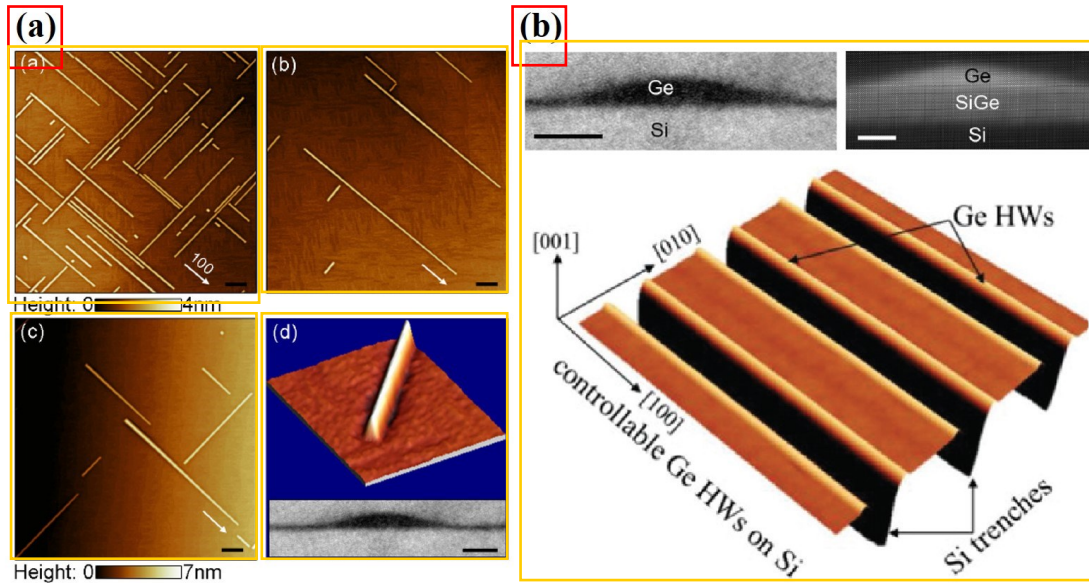
图 1.7 (a) 棚顶型 Ge 纳米示意图，图片引自[35]。(b) 位置可控的棚顶型 Ge 纳米示意图，图片引自[36]。
