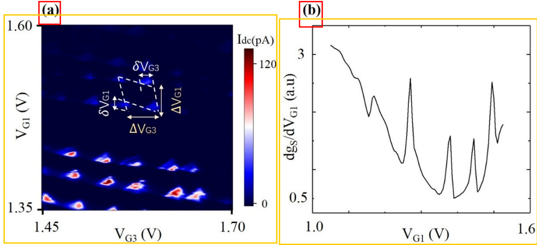
图 5.4 (a) V_{SD} = 2 \text{ mV} , V_{G2} = 1.2 \text{ V} ，双量子点直流输运的电荷稳定性相图。(b) 空穴在双量子点之间运输时，会引起电荷感应器的电导变化从而观测到微分电导峰。
