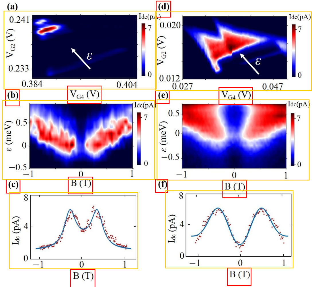
图 3.5(a) 在 V_{SD} = 2.5 \text{ mV} ， V_{G1} = 0.44 \text{ V} ， V_{G3} = -0.02 \text{ V} ， V_{G5} = -0.015 \text{ V} 时观测到的自旋阻塞区域，白色箭头为沿着失谐量 \varepsilon 的方向。(b) 图(a)中自旋阻塞区域漏电流随外加磁场及失谐量 \varepsilon 演化的图像。(c) 提取图(b)中 \varepsilon = 0 处漏电流的数据（红色圆点）并进行拟合（蓝色实线），漏电流的线型呈现出在零磁场附近为谷的双峰结构。(d) 双量子点中的空穴数增加，测量到另外一个自旋阻塞区域。(e) 图(d)中自旋阻塞区域漏电流随外加磁场和失谐量 \varepsilon 演化的图像。(f) 提取图(e)中 \varepsilon = 0 处漏电流的数据（红色圆点）并进行拟合（蓝色实线），漏电流的线型呈现出更宽的双峰结构。
