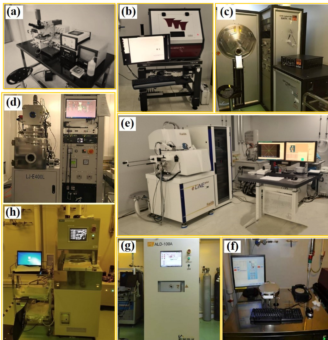
图 2.5 微纳加工常用仪器设备：(a) MJB3 型紫外光刻机。(b) Microwriter ML3 激光直写光刻机。(c) MARK-40 电子束蒸发镀膜机。(d) LJ-E400L 电子束蒸发镀膜机。(e) E-line 电子束曝光机。(f) 热型原子层沉积仪器 Thermal-ALD。(g) 等离子体原子层沉积仪器 PE-ALD。(h) 反应离子刻蚀机。
