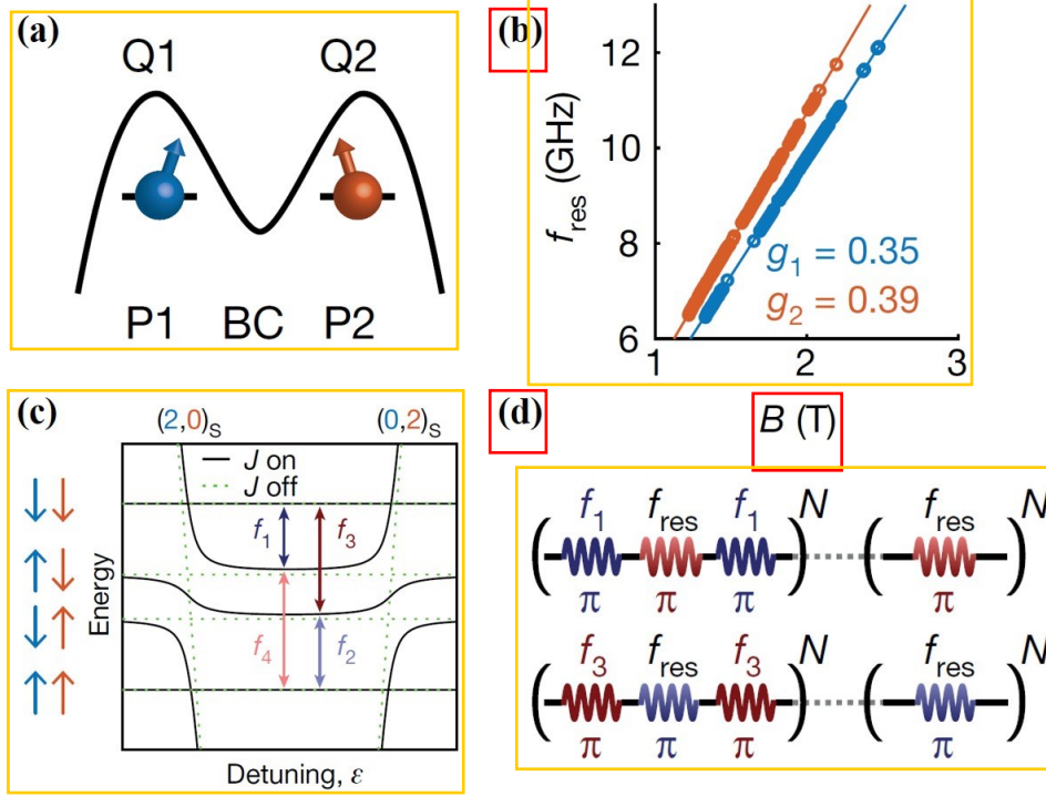
图 6.1 (a) 双量子点中两比特示意图。(b) 两个空穴的自旋都发生翻转时，观测到两条斜率不同的电偶极自旋共振谱线。(c) 两比特不同自旋态的能级，可以通过交换作用能 J 进行调节。(d) 不同频率的微波脉冲序列示意图。图片引自[4]。
