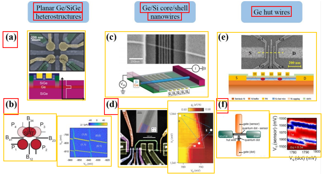
图 1.8 (a)和(b) Ge/SiGe 平面异质结四量子点结构示意图，并基于此结构实现了 RF 电荷探测，图片引自[38]。(c) Ge/Si 核壳纳米线三量子点结构示意图，图片引自[40]。(d) Ge/Si 核壳纳米线双量子点，并集成电荷感应器来探测空穴的自旋弛豫，图片引自[41]。(e) 栅顶型 Ge 纳米线双量子点结构示意图，图片引自[48]。(f) 基于栅顶型 Ge 纳米线的 RF 探测器，图片引自[47]。
