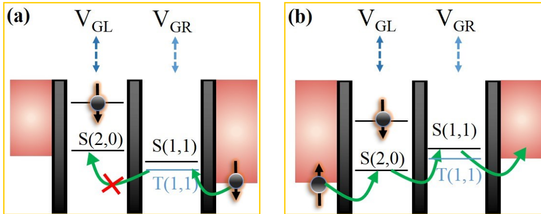
图 1.4 (a) 双量子点中泡利自旋阻塞示意图。当 QD_L 中已经占据了一个自旋向下的空穴时，由于自旋不相容原理， QD_R 中同样自旋向下的空穴不能从 T(1,1) 态隧穿到 S(2,0) 态。(b) 当源漏偏压反向时，自旋向上的空穴时可以从 QD_L 中 S(2,0) 态输运到 QD_R 中的 S(1,1) 态，泡利自旋阻塞被解除。
